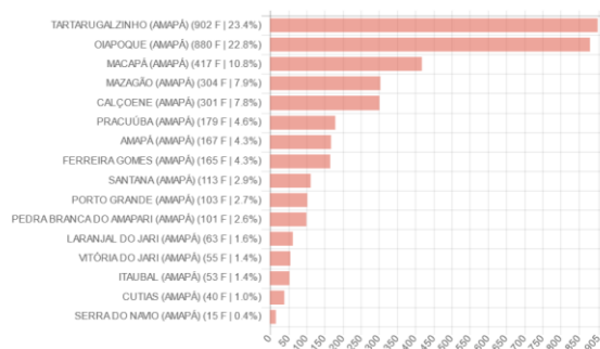
FOCOS POR MUNICÍPIO (3858 FOCOS, DE 2023/10/01 A 2023/10/08)
